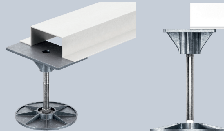
Anwendungsmöglichkeit 1 – Aluminium-Stelzlager
