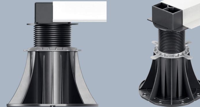
Anwendungsmöglichkeit PP-Stelzlager
